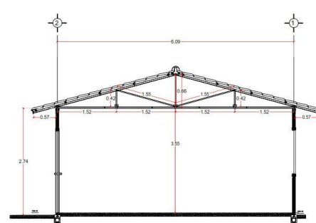
CORTE TRANSVERSAL
