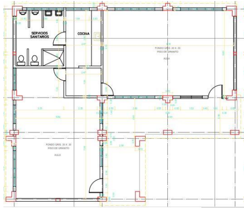
MODULO DE 2 AULAS ARTICULADO
