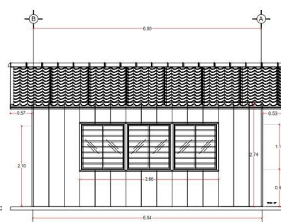
FACHADA POSTERIOR
