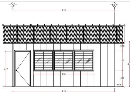
FACHADA FRONTAL
