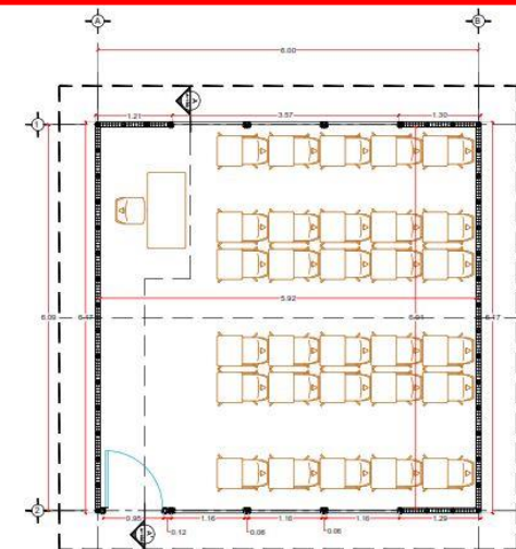
PLANTA ARQUITECTONICA
